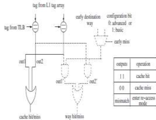
FIG.4. Way Hit/Miss Decoder
